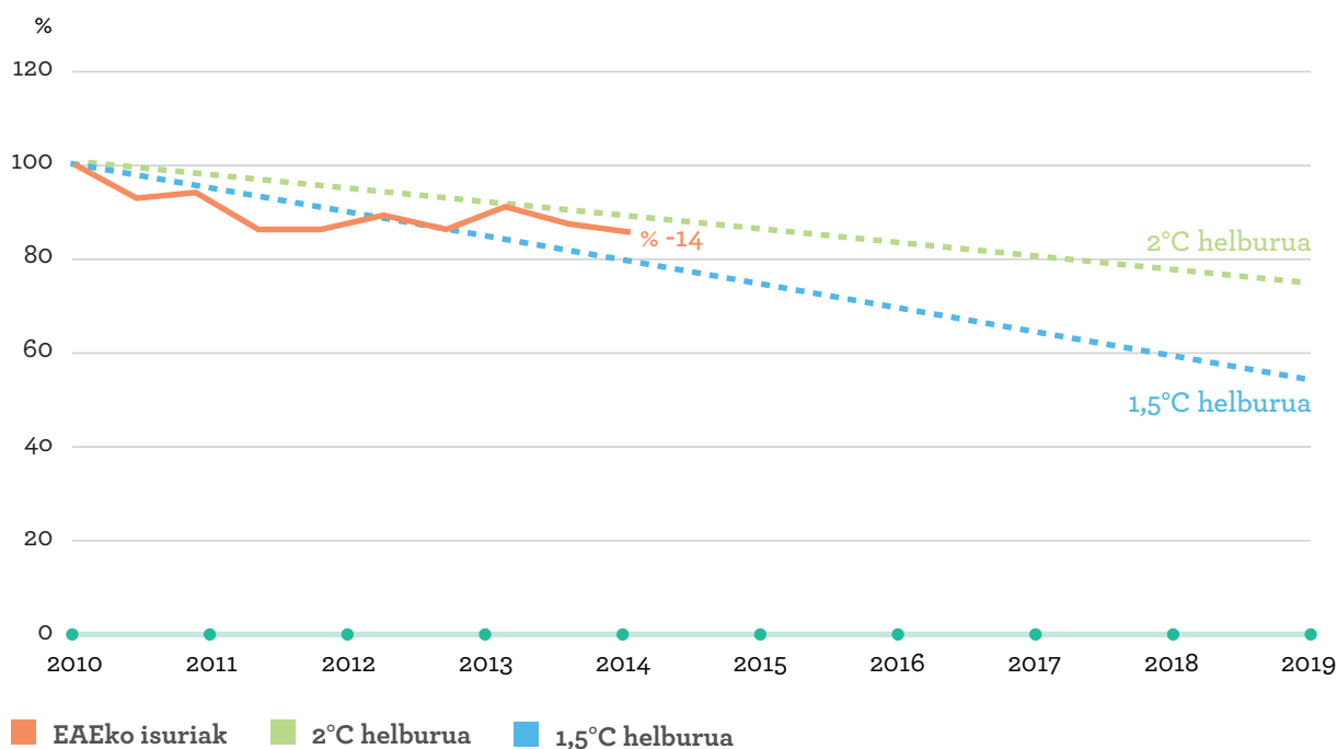
Isurien bilakaera versus IPCC 1,5 °C txostenaren helburuak (2010 = 100)
